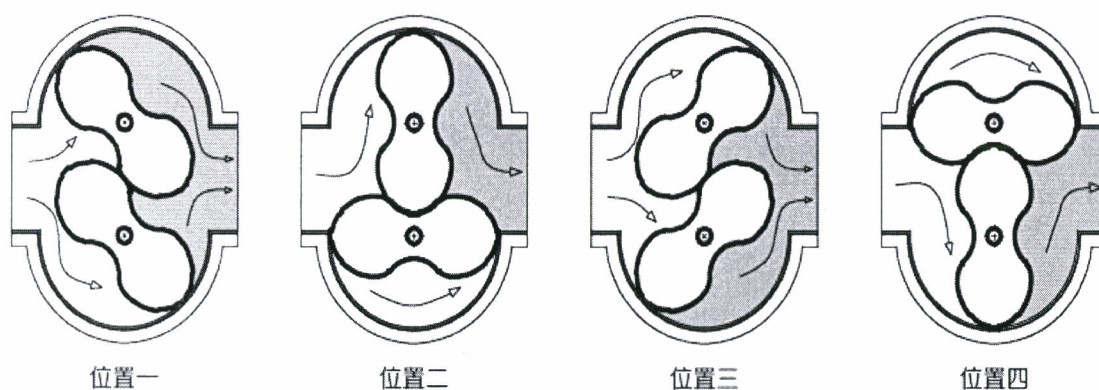
图 2 罗茨（腰轮）流量计的工作原理图
